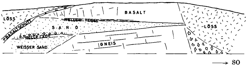
Abb. 4. Schematische Ansicht der Straßenaufschlüsse südlich des Basaltsteinbruchs von Stob. (Die stellenweise ganz aussetzende rote Lehmlage zwischen dem hellen [sandigen] Tegel und dem Basalt ist nicht besonders ausgeschieden.)
